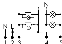
instalacja 4-przewodowa
